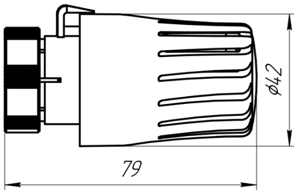
Рисунок 1 – Габаритные размеры
